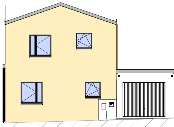
Facade Nord
