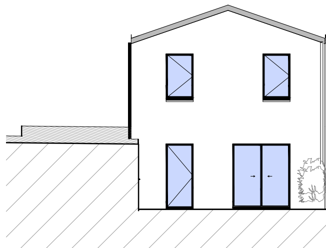
Facade Est
