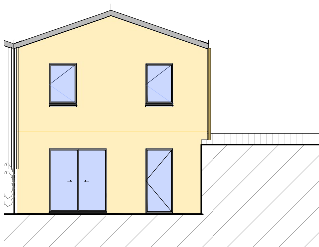
Facade Est
