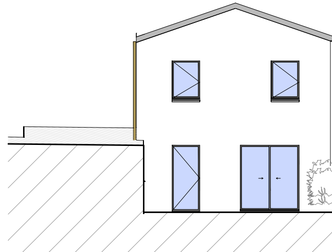
Facade Est
