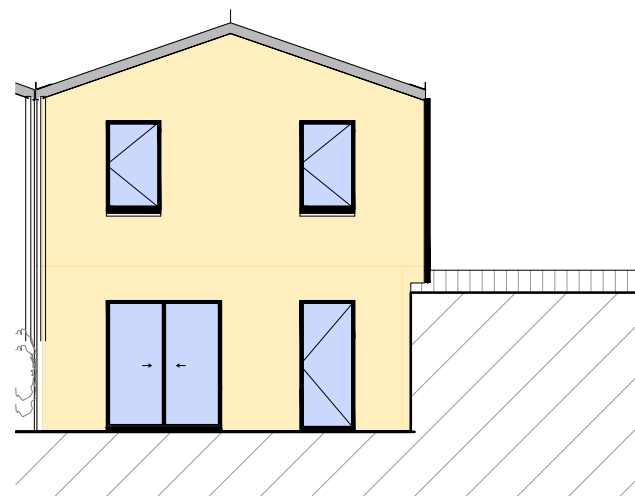
Facade Est
