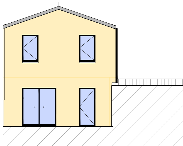
Facade Ouest
